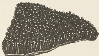
MANGANESE ORE.
